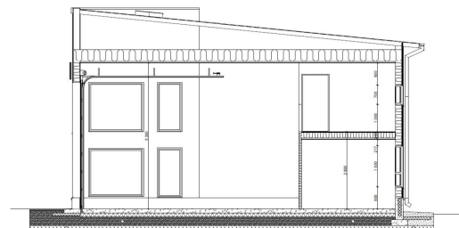
Leikkauskuva
